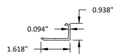
34 1" X 1 11/16" CLIP
